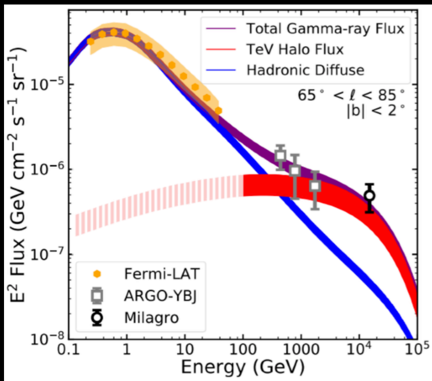
Diffuse TeV Flux
